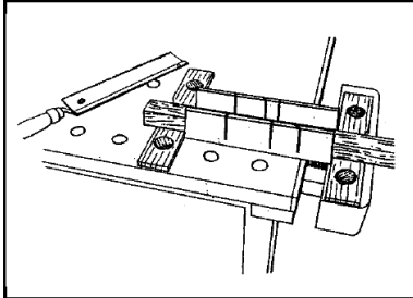
Sägen mit Gehrungsschneidladen
