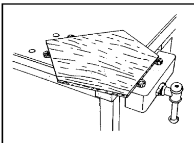
Einspannen unförmiger Werkstücke
